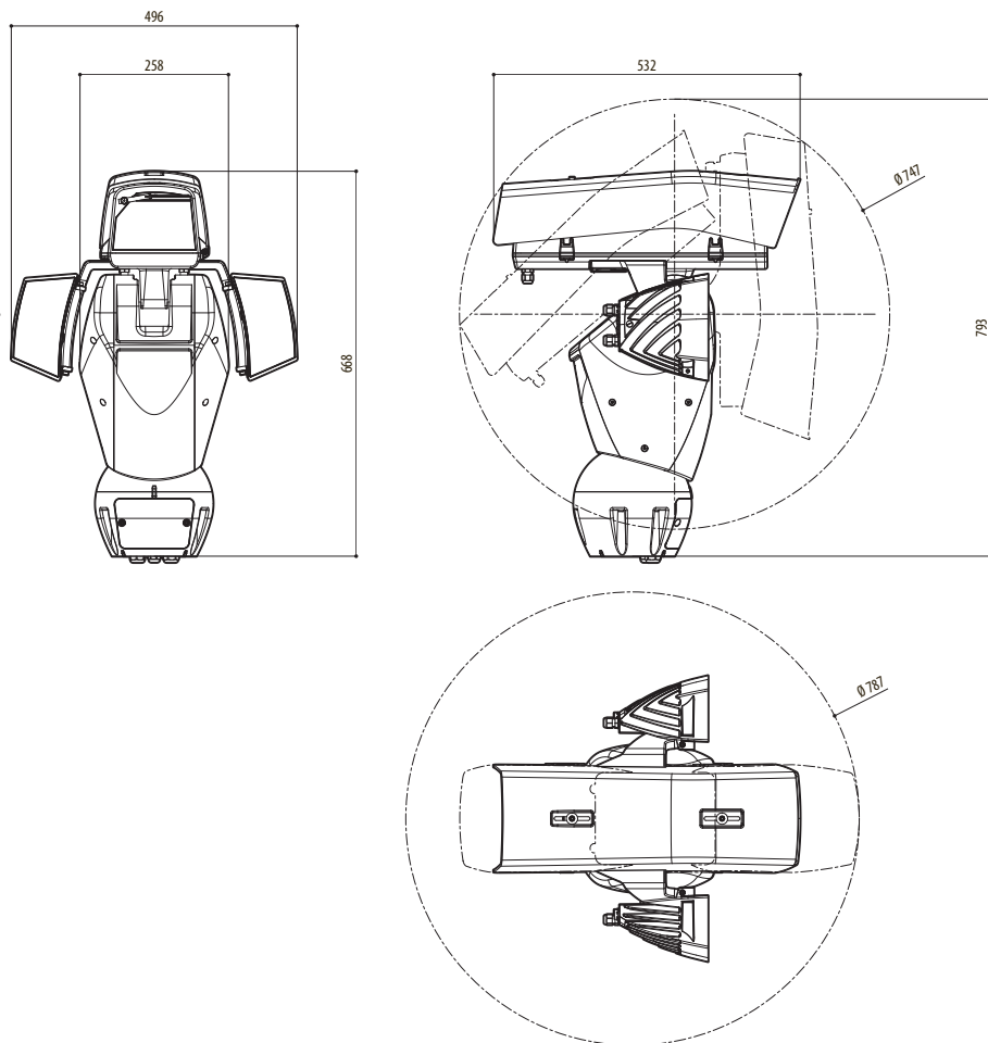
Fig. 111 ULISSE2, version avec 2 projecteurs à LED.
