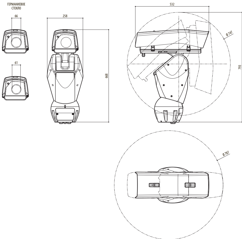
Рис. 112 ULISSE2, модель для тепловизоров.
