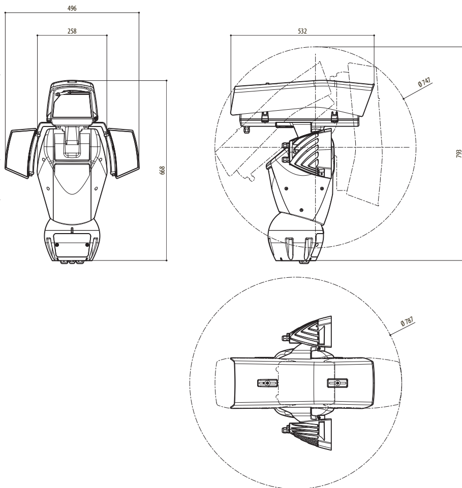
Рис. 111 ULISSE2, версия с двумя светодиодными осветителями.
