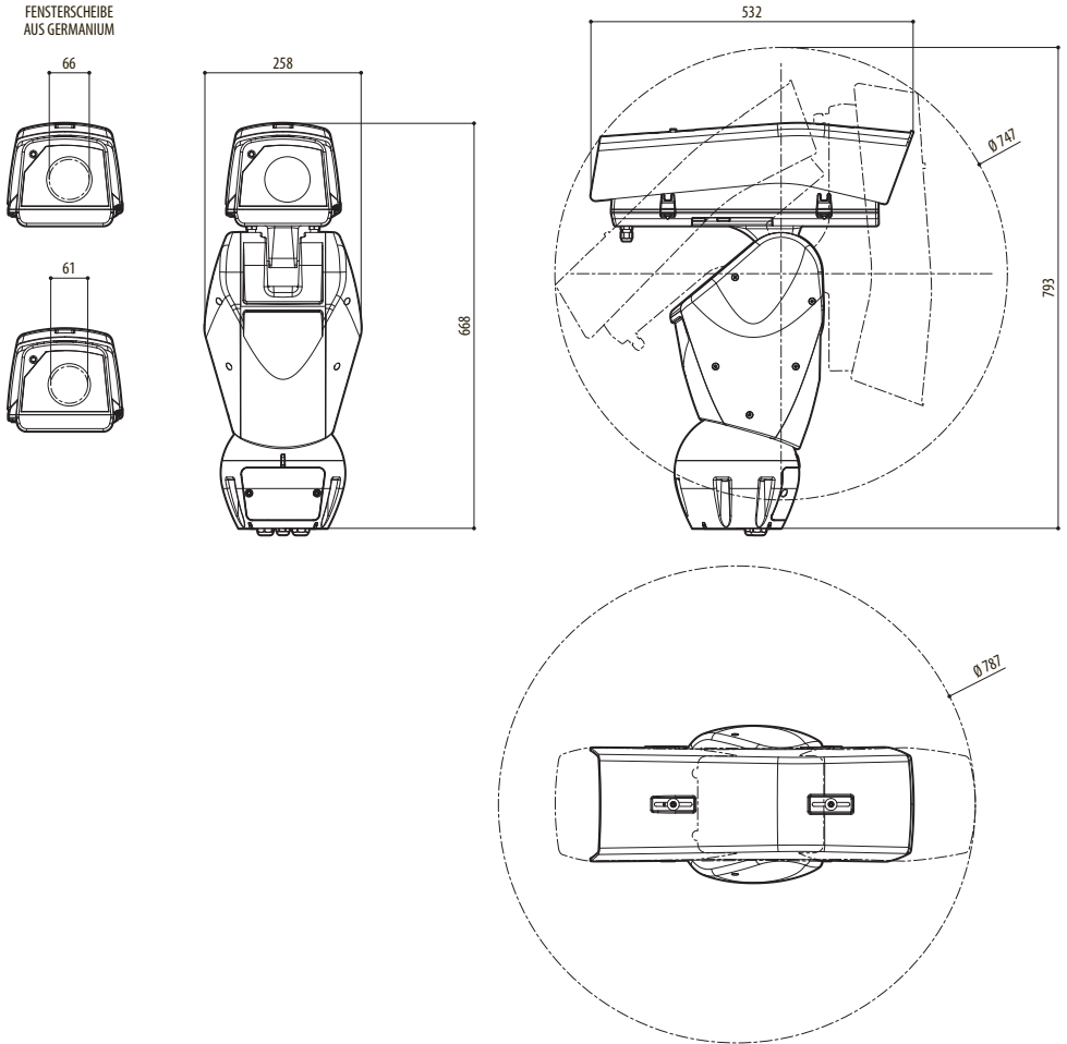
Abb. 112 ULISSE2, Version für Wärmebildkameras.
