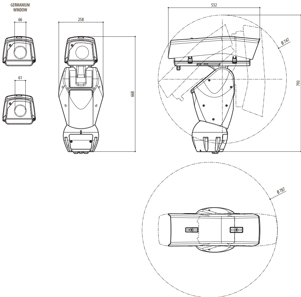
Fig. 112 ULISSE2, version for thermal cameras.
