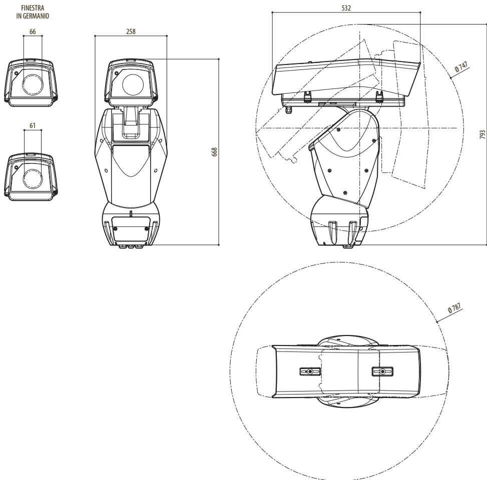
Fig. 112 ULISSE2, versione per telecamere termiche.
