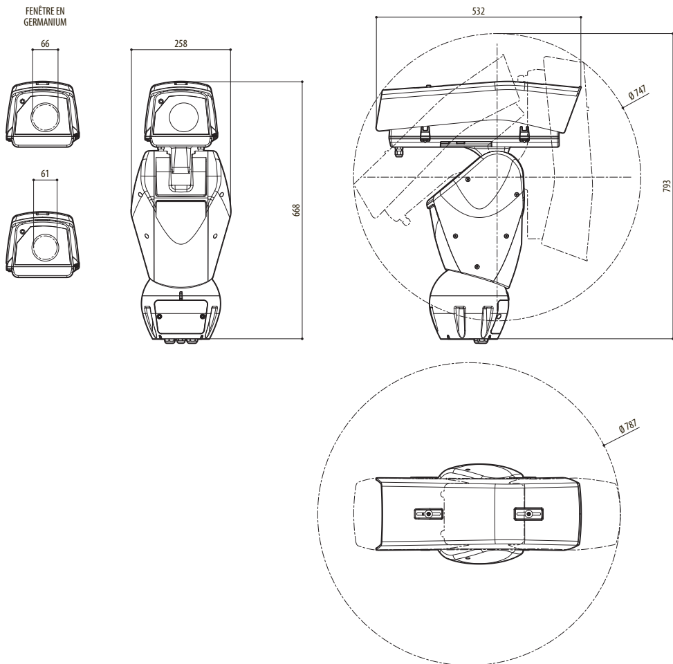
Fig. 112 ULISSE2, version pour caméras thermiques.
