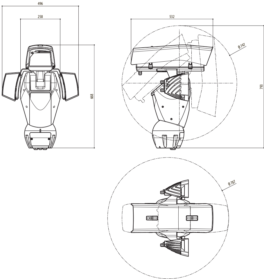
Abb. 111 ULISSE2, Ausführung mit zwei LED-Scheinwerfern.
