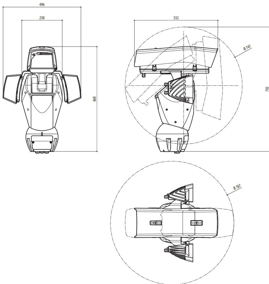
Fig. 111 ULISSE2, versione con due illuminatori a LED.
