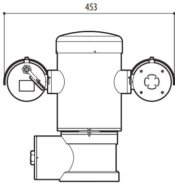
Fig. 139 MAXIMUS MPXT.
