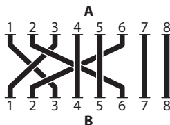
Fig. 28 Câble sertissé.
