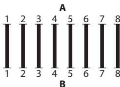
Fig. 27 Câble croisé.
