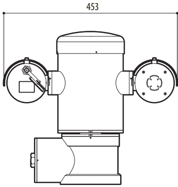
Abb. 139 MAXIMUS MPXT.
