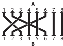
Рис. 28 Перекрёстный кабель.
