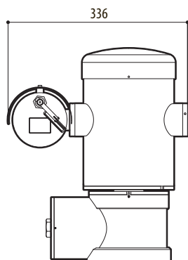
Рис. 138 MAXIMUS MPX.
