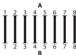
Рис. 27 Прямой кабель.
