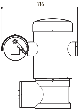
Abb. 138 MAXIMUS MPX.
