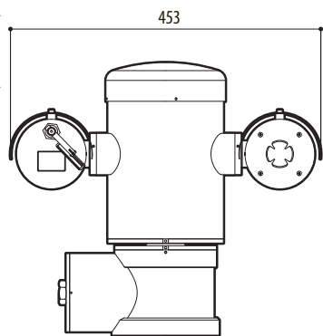
Рис. 139 MAXIMUS MPXT.
