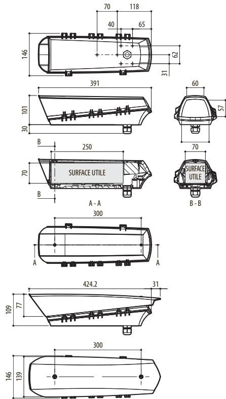
Fig. 14 PUNTO Hi-PoE.
