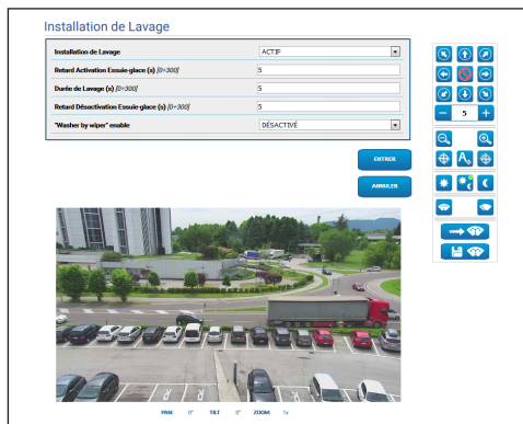
Fig. 60 Page-écran PTZ
