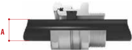
Kabeldurchführung mit Gummidichtung mit nicht armiertem Kabel
