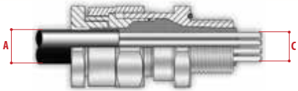
Kabeldurchführung mit Dichtbarriere mit nicht armiertem Kabel
