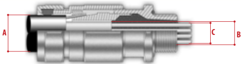
Kabeldurchführung mit Dichtbarriere mit armiertem Kabel
